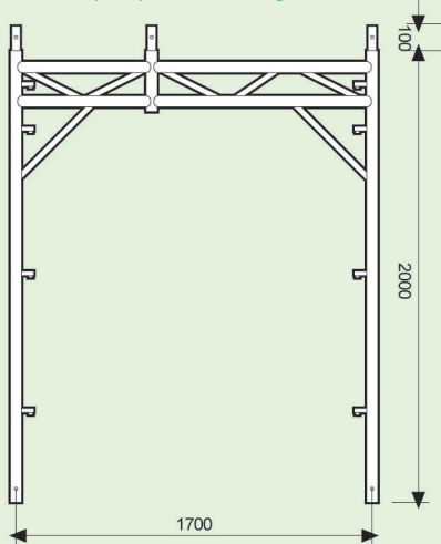
Telaio per partenza larga 1700
