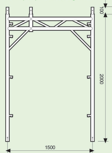
Telaio per partenza larga 1500
