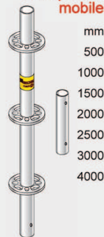
Montante con spinotto mobile
