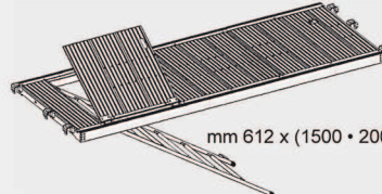
Tavola palco in alluminio con angoli mobili
