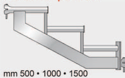
Fianco rampa scala
